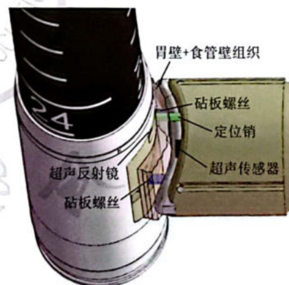
图2 MUSE 内镜结构原理图
